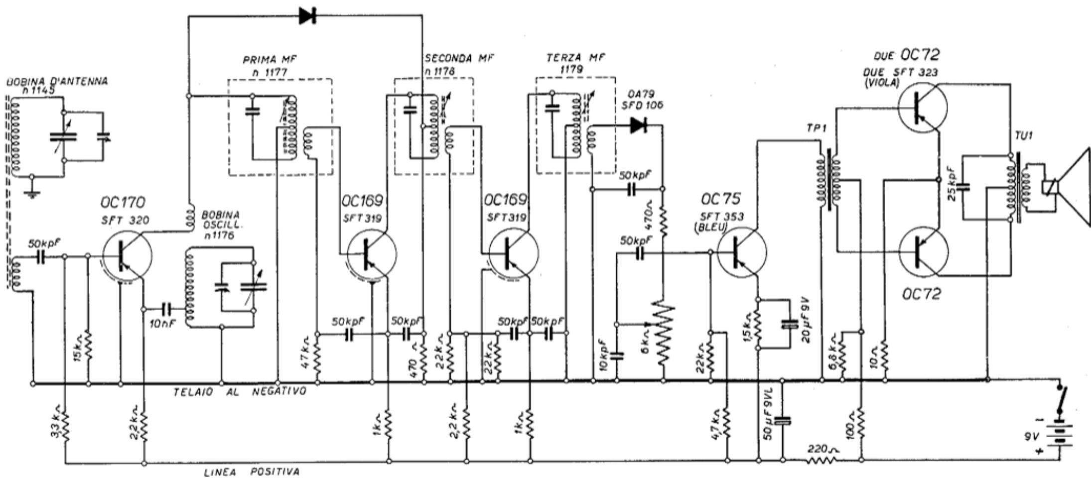
Geloso G3303 Polaris
